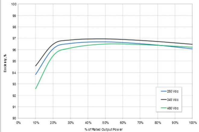
PVI-6000-TL-OUTD
